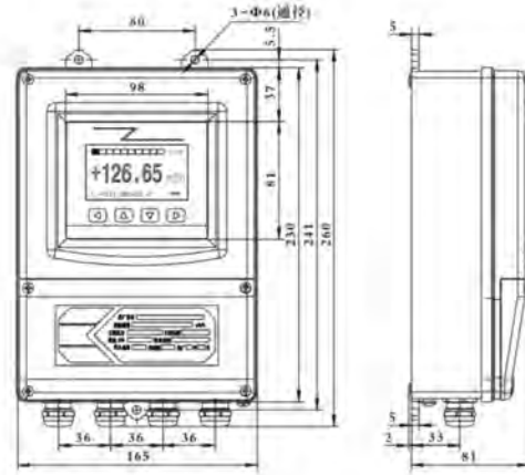
智能转换显示器外形图
