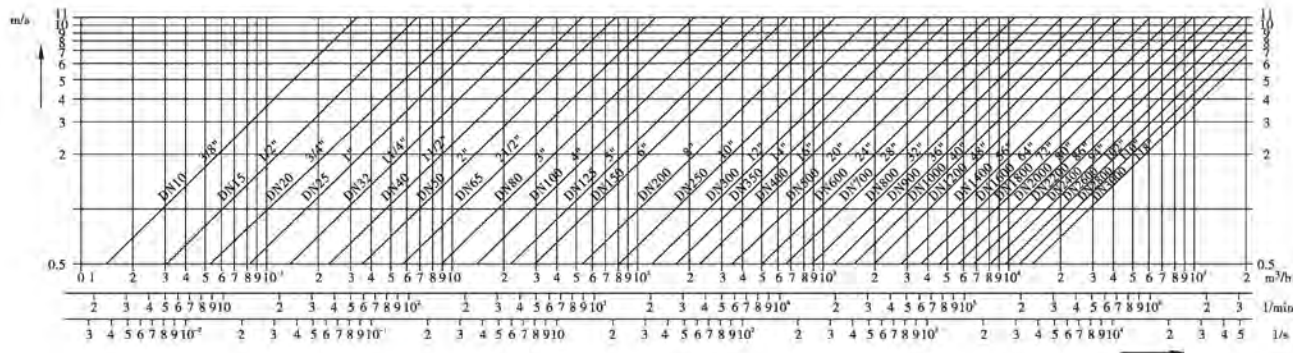
流量计口径、流速与流量关系曲线图
