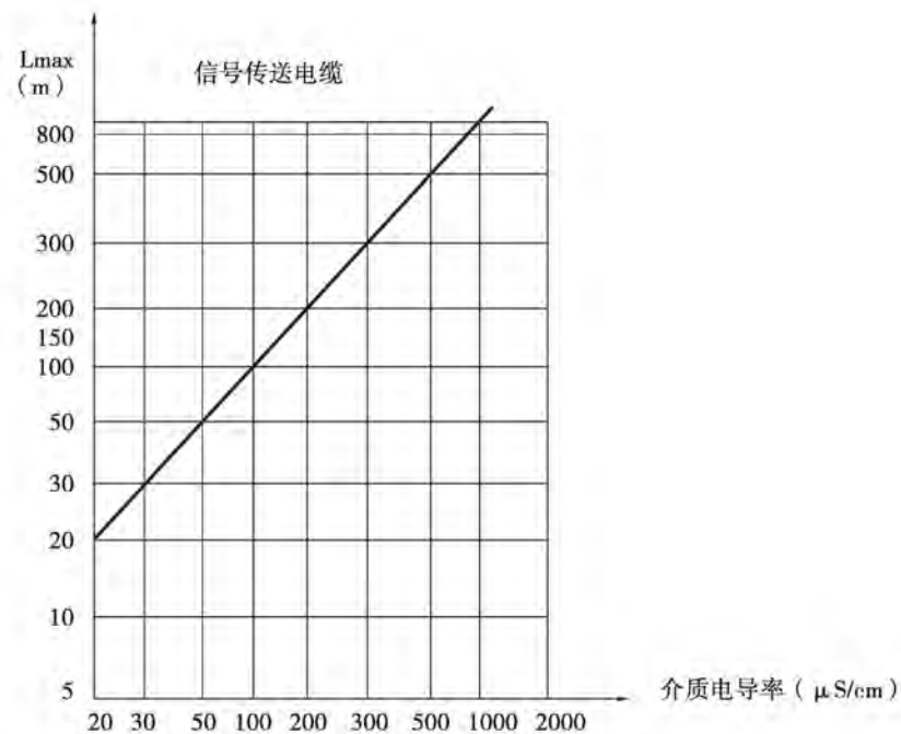
分体式最大距离、电缆铜芯截面与介质电导率关系曲线图
