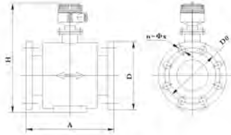
分体型传感器外形图
